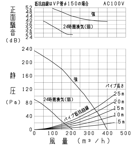
VD-20ZLC 13 -IN/P-Q・騒音特性
