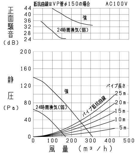
VD-18ZLC 13 -IN/P-Q・騒音特性
