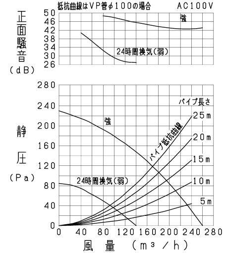
VD-18ZLSC 13 -IN/P-Q・騒音特性
